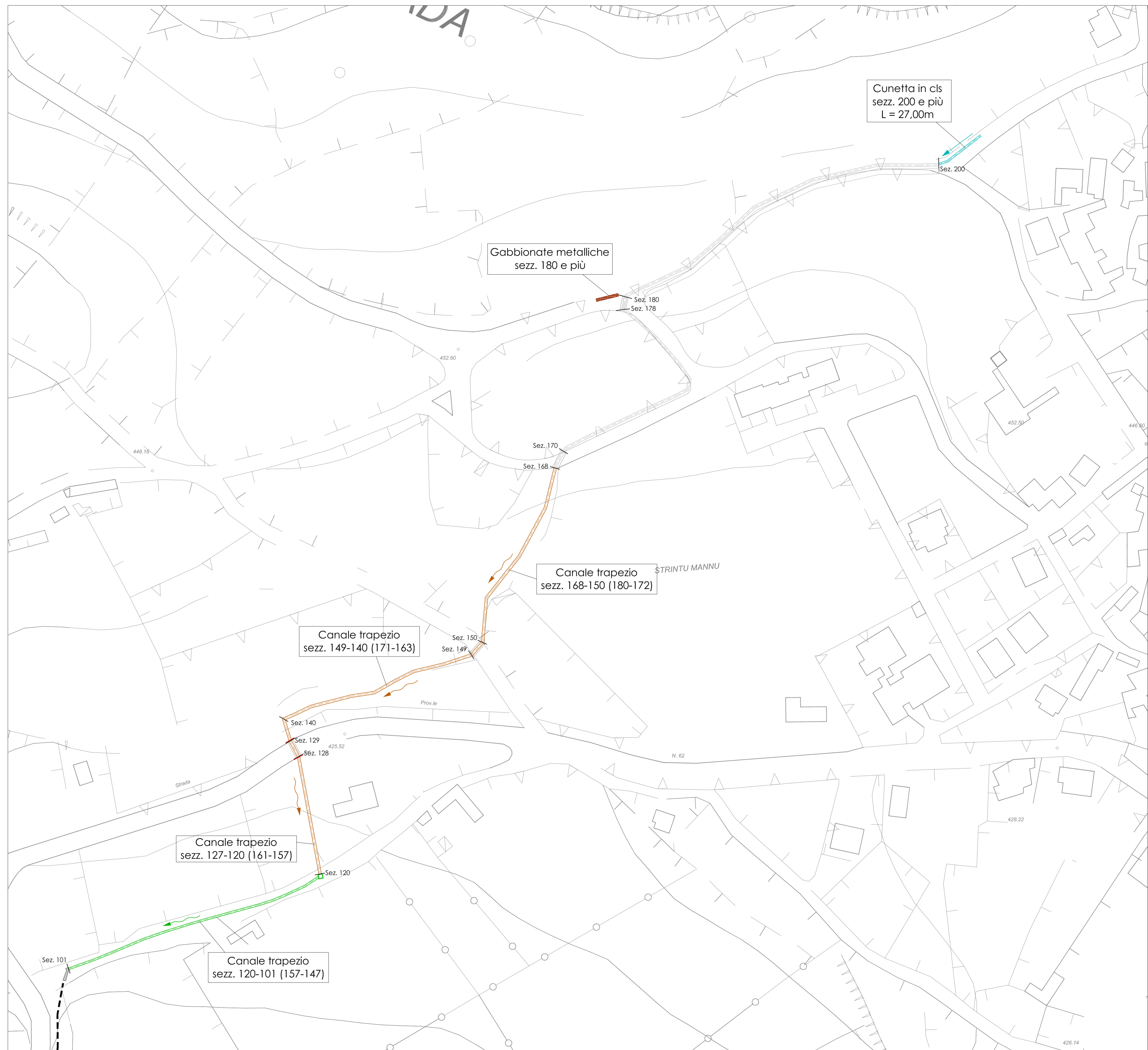
PLANIMETRIA OPERE IN PROGETTO
